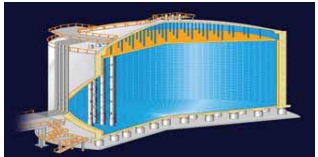
LNG Terminal Tank Insulation
